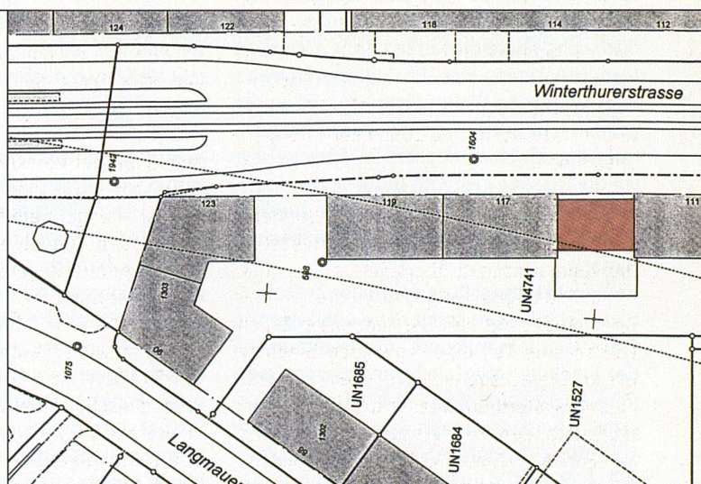
Situation der Siedlung Langmauer-/ Winterthurerstrasse im Zürcher Kreis 6 mit neuem Zwischenbau.
