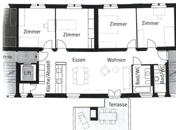
Grundriss einer 5 1/2-Zimmer-Wohnung mit 121 Quadratmetern Wohnfläche und 15-Quadratmeter-Terrasse. Wegen der Zusammenlegung verfügen die neuen Grosswohnungen über zwei Eingänge.
