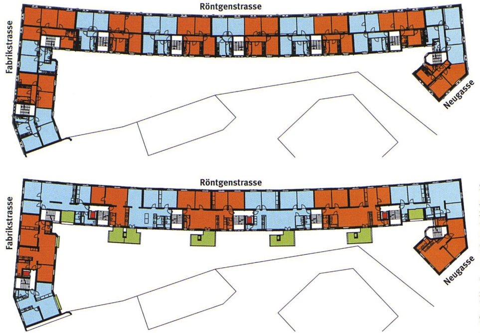
Grundrisse alt und neu (1. OG): Jeweils zwei Wohnungen wurden zusammengelegt. Dabei blieb die Schicht gegen die Strassenseite meist unverändert, während gegen die Hofseite grosse Wohn-Ess-Zimmer mit individuellen Aussenräumen entstanden.
