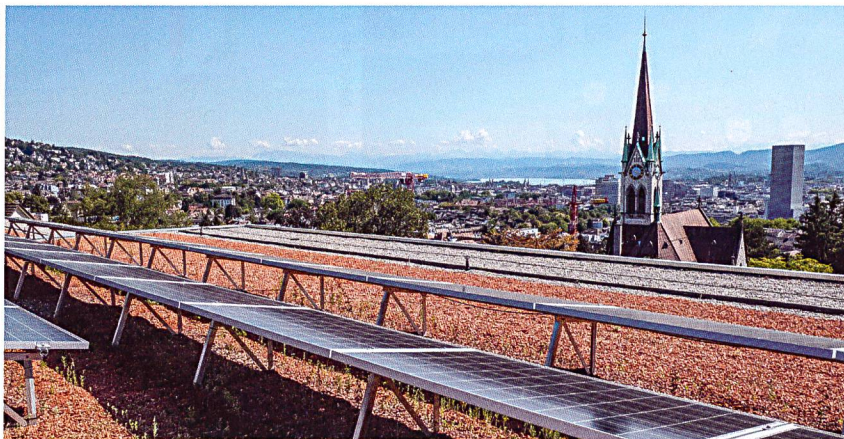
Alle Dächer sind mit PV-Anlagen ausgestattet, die Strom für die Wärmepumpen und die Bewohner liefern. Auf einem Haus erzeugen PVT-Hybridkollektoren zusätzlich Wärme zur Regeneration der Erdsonden.
