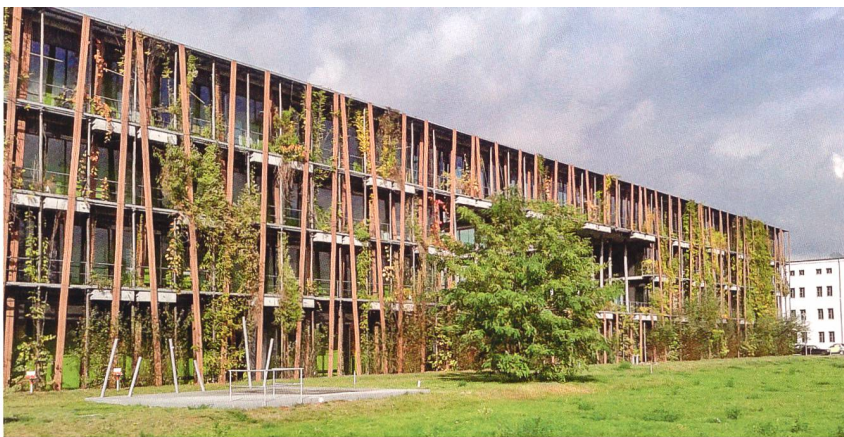
1 Eine gelungene Mischform aus bodengebundener und fassadengebundener Begrünung in Trögen findet sich bei der Humboldt-Universität zu Berlin in Adlershof. Die Pflanzen unterstützen den sommerlichen Wärmeschutz.
