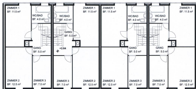
Obergeschoss
