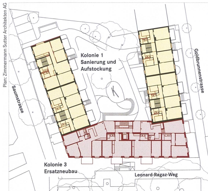
Der Ersatzneubau fügt sich passgenau allseitig in den Blockrand ein. Das zentrale Element ist das hofseitige, gemeinschaftliche Treppenhaus, über das vier Wohnungen pro Geschoss erschlossen sind.
