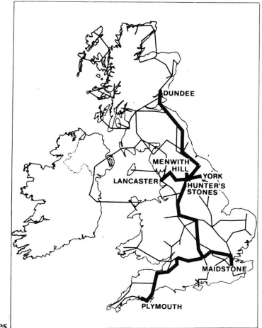
Hunters Stone ist das Zentrum des Britischen Mikrowellenübertragungsnetzes
