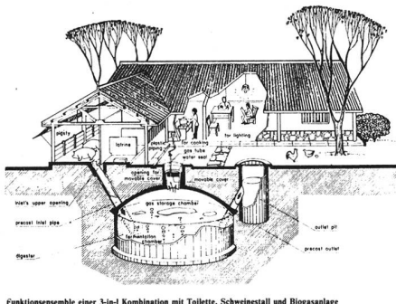
Funktionsensemble einer 3-in-1 Kombination mit Toilette, Schweinstall und Biogasanlage
