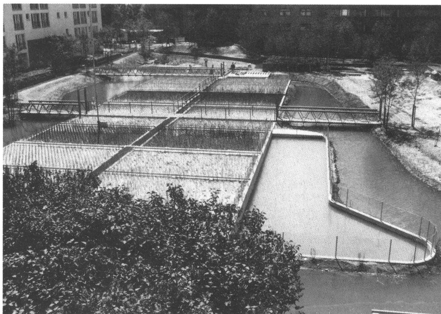
Außenanlage des integrierten Wasserkonzeptes (im Bauzustand kurz nach der Bepflanzung): In der Mitte ist die mit Schilf und Binsen bepflanzte Kläranlage erkennbar, an die sich rechts der sogenannte Schönungsteich zur Nachklärung anschließt. Umgeben wird die Anlage von einem 1000 m 2 großen Regenwasserteich. Das in den Wohnungen getrennte Grau- und Fäkalwasser wird in die insgesamt vier Module eingeleitet, nachdem ihm ein Teil der Wärme entzogen wurde. Die Sumpfpflanzen sind über ihre Wurzeln in der Lage, die zum biologischen Abbau verantwortlichen Bakterien mit Sauerstoff zu versorgen.
