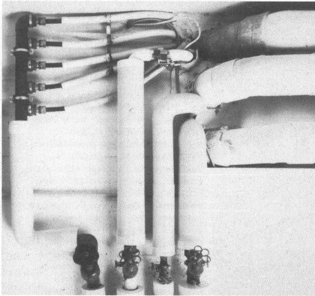
Rechts befinden sich die Abwasserleitungen für Regen-, Grau- und Fäkalwasser; im Vordergrund die Trinkwasserleitungen; links davon die Betriebswasserleitungen (gereinigtes Abwasser aus der Pflanzenkläranlage z.B. zur Versorgung der Toilette)
