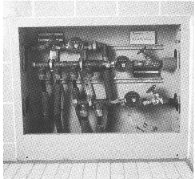
Verteilungssystem in der Wohnung: Der mittlere Verteiler versorgt z.B. die Badewanne mit (kaltem) Trinkwasser; der untere führt warmes Trinkwasser, der obere Betriebswasser für die Toilette. Durch das Rohr-in-Rohr-System kann – ohne in die bauliche Substanz eingreifen zu müssen – z.B. später die Waschmaschine mit Regenwasser versorgt werden.
