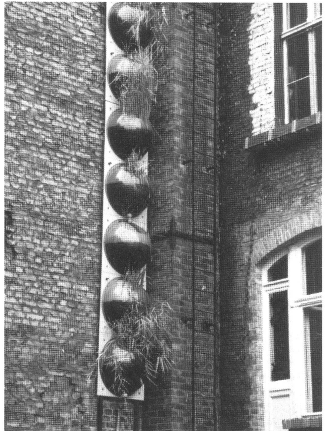
Vertikalsumpf im Altbau: In den Behältern wachsen Schilf und Binsen als Substrat dient Blähton. Das Grauwasser wird in den obersten Behältern gepumpt und fließt im freien Fall von einem zum nächsten nach unten.
