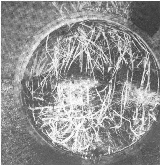
Durch die Wurzeln der Binsen und des Schilfs im Vertikalsumpf wird das Wasser gereinigt und kann anschließend als gereinigtes Grauwasser z.B. für die Toilettenspülung als Trinkwassersubstitution eingesetzt werden.
