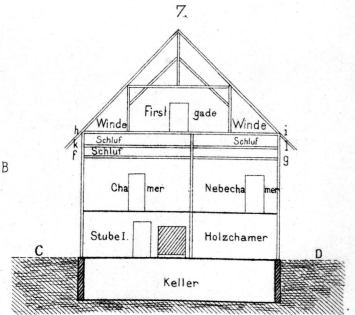
Querdurchschnitt 1:200
