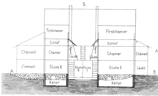
Längendurchschnitt 1:200
