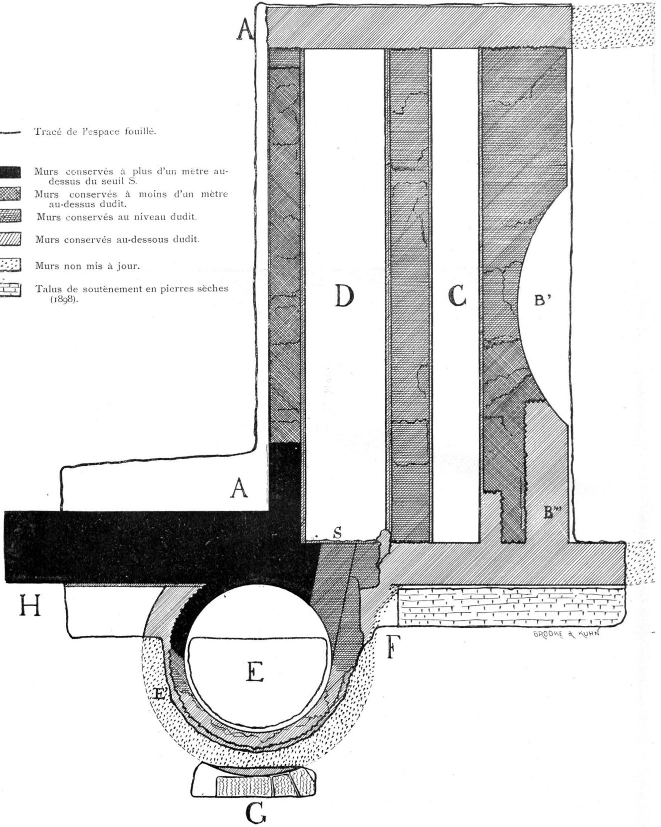
AVEN PLAN DE LA PORTE DE L'EST D INDICATEUR D'ANTI
