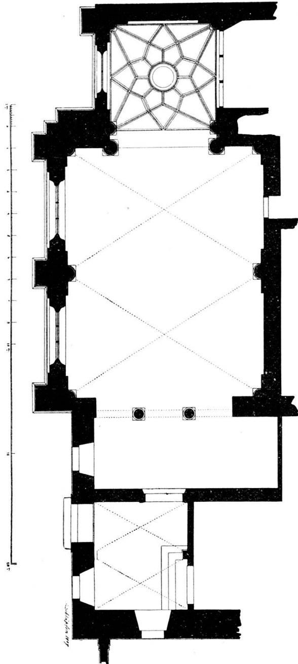
31. Kirche der Ursulinerinnen in Freiburg. Aufnahme von K. Schlöpfer. M = 1:200.
