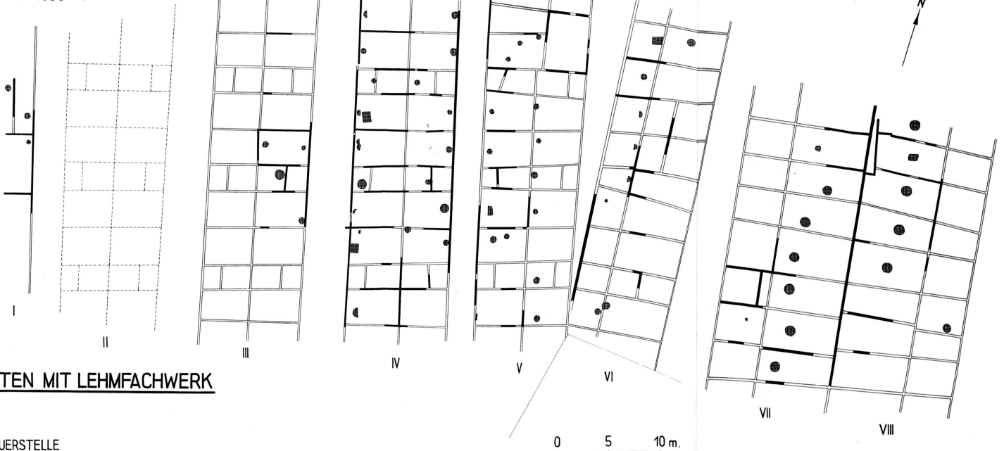
Abb. 5. Die Bauten mit Lehmfachwerk der 3. Per.
