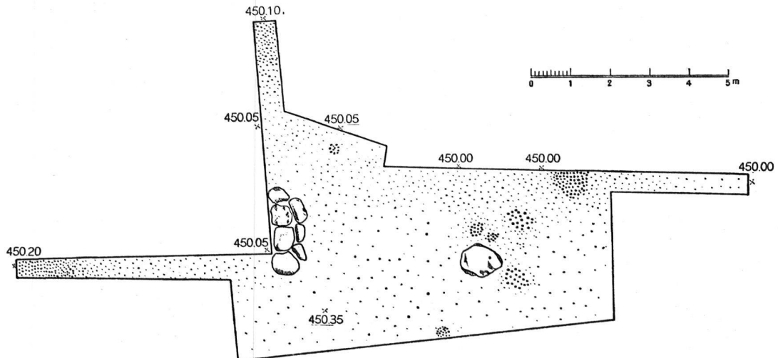
Abb. 4. Herblingen/Grüthalde: Grundriß-Plan der Grabungen 1938/39, erstellt vom Vermessungsamt des Kantons Schaffhausen (Kantonsgeometer H. Bührer) mit Einzeichnungen des Verfassers
