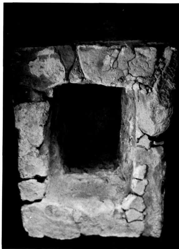
a–e Blockaltar in der Kirche St. Lorenz bei Paspels (vgl. dazu auch Abb. 6): a Zustand vor Entfernung der barocken Anmauerungen (an der Basis), b Mensaplatte (vgl. dazu auch Abb. 7), c Zustand des Altars nach Abheben der Mensaplatte, d Altar nach Durchschlagen der Weisskalkschicht, e Inneres des (entleerten) Altars.
