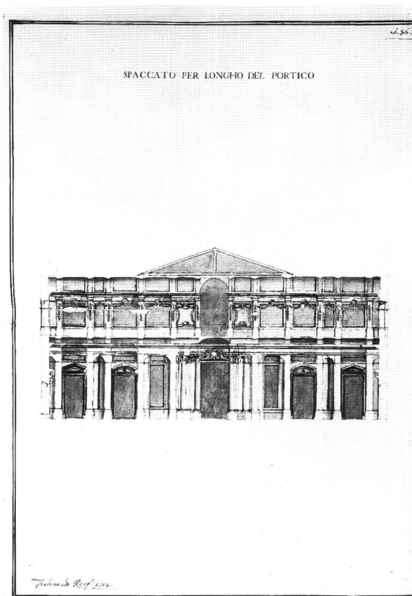
Fig. 6 Façade pour la basilique Saint-Jean de Latran, coupe longitudinale, de Ferdinando Reyff, 1705. Dessin à l'encre de chine et à l'aquarelle, 80 × 74 cm.
