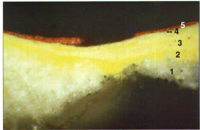
Abb. 20 Karton IV, Querschliff vom linken Bein des Hellebardiers (Probe Nr. 51). Abfolge: Fasern vom Träger (0); grundierungsartige weisse Farbe (Calcitmehl, Protein) (1); darauf nass in gelber Farbschicht (2); hellgelbe Übermalung: Gewandfarbe (Strontiumgelb, Bleiweiss, Baryt in Öl) (3); weisse Lasur (4); dünne hellrote Farbschicht: Gemalte Blutspur (5). Mikroskopisches Bild im Auflicht, Bildbreite = 0,79 mm.
