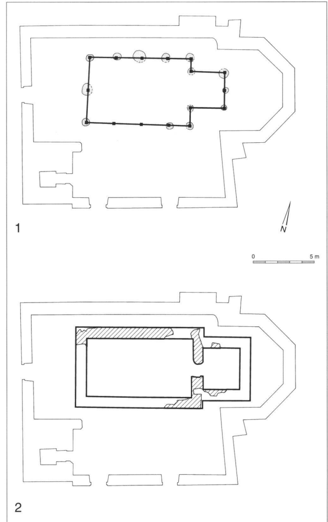
Abb. 6 Oberwil bei Büren a.A., ehemals St. Maria. 1 Erste Holzkirche mit Rechteckchor, 8. Jahrhundert. Es bleibt offen, ob die erste Kirche nicht durch einen Saal gebildet wurde, an den man erst nachträglich das Rechteckchor ansetzte. 2 Erste Steinkirche, 9./10. Jahrhundert.
