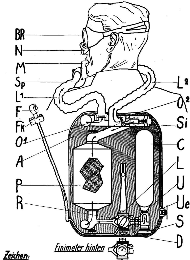
Abb. 2. Schematische Darstellung der Wirkungsweise des Sauerstoff-Gaschutzgerätes Dräger Type KG 130.
