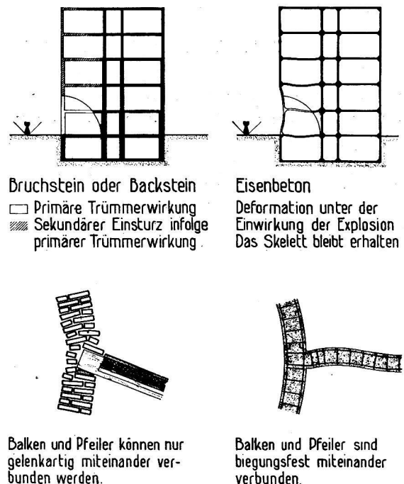
Abb. 17. Schematische Darstellung.
