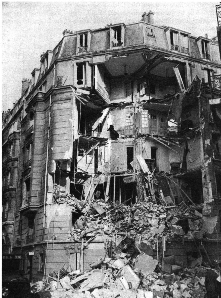
Abb. 12. Halb zerstörtes Haus. Der Rand der Zerstörung zeigt die gleiche birnförmige Linie, wie das Spannungsdiagramm in Abb. 11. Diese Ausbauchung zeichnet sich links und rechts, sowie auch in der Tiefe ab. Fast die ganze Fassade hat es gegen den Sprengherd zugeworfen. In den Trümmern vor dem Haus erkennt man Teile des Dachgesimses. Im Hausinnern liegen nur die Böden und Innenmauern. Der Schuttkegel vor dem Haus ist nur etwa 2 m hoch. Der Sog hat alle Türen gegen den Explosionsherd hin geöffnet.
