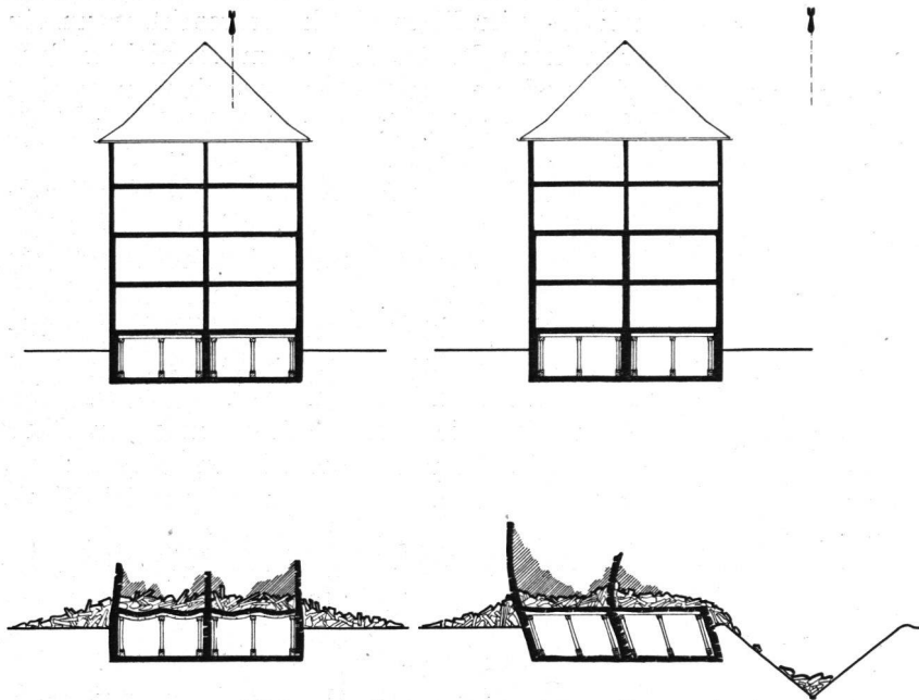
Abb. 15. Schematische Darstellung.
