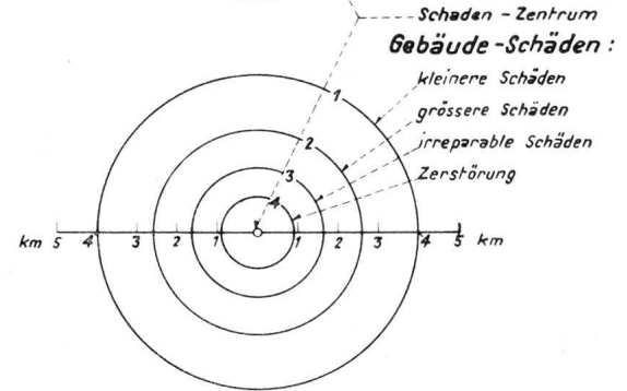
Abb. 23. Englischs Schema mit den Wirkungsradii der 20-kt-Bombe mit hohem Sprengpunkt, auf Grund der Beobachtungen in Hiroshima und Nagasaki. Die im unteren Diagramm dargestellten Kreise beziehen sich auf Gebäude europäischer Bauart. (Nach dem Diagramm in «Report of the British Mission to Japan», London 1946.)
