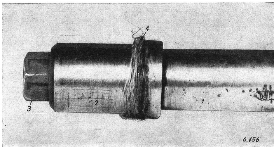
Abb. 9. Dichtung aus Hanf statt aus weichem Gummi. 1 Mischrohr, 2 Schaft, 3 Injektordüse, 4 Hanf.
