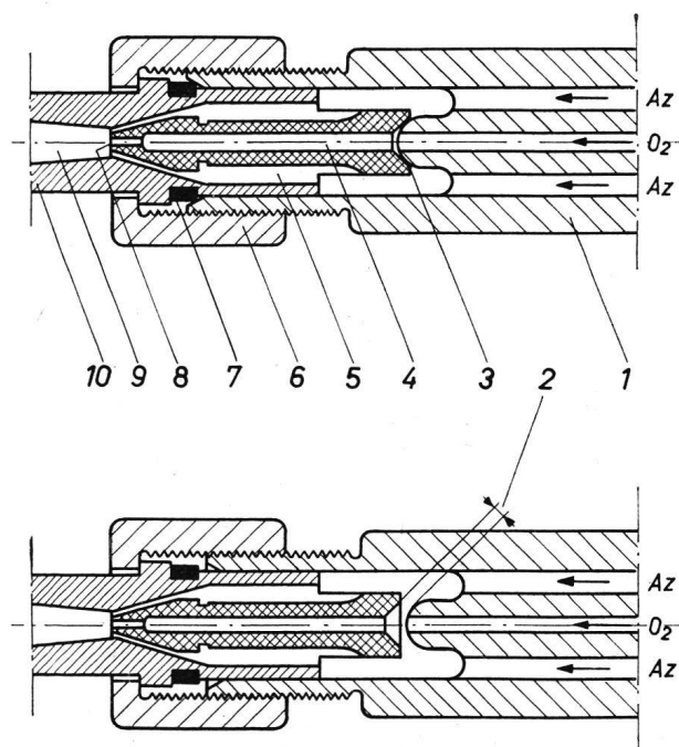
Abb. 7. Verbindung von Brennerhandgriff und Einsatz. Ordnungsgemäss zusammengesetzter Brenner. 1 Handgriff, 2 Spalt, 3 innere Dichtungsfläche, 4 Sauerstoffkanal des Injektors, 5 Azetylenkanal, 6 Ueberwurfmutter, 7 Gummidichtung, 8 Sauerstoffmündung der Injektordüse, 9 Mischrohr, 10 Brenneinsatz.
