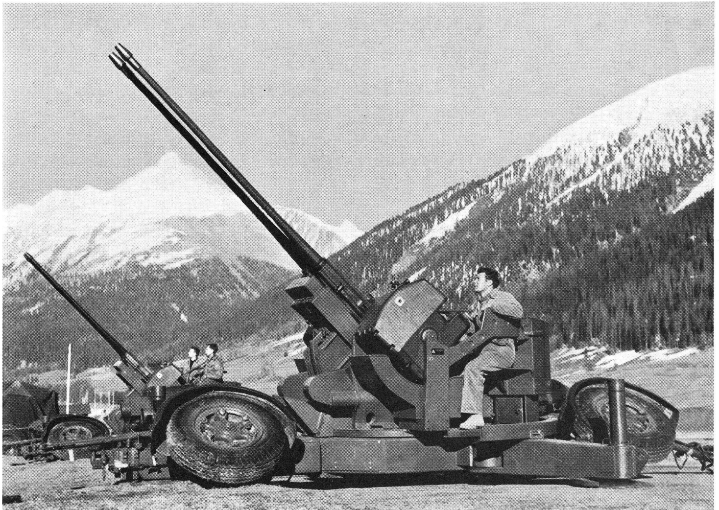
Zwei 35-mm-Zwillings-Geschütze Oerlikon-Contraves in Feuerstellung
