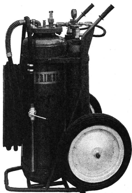
PRIMUS Luftschaum-Feuerlöschgerät Typ LS 75
