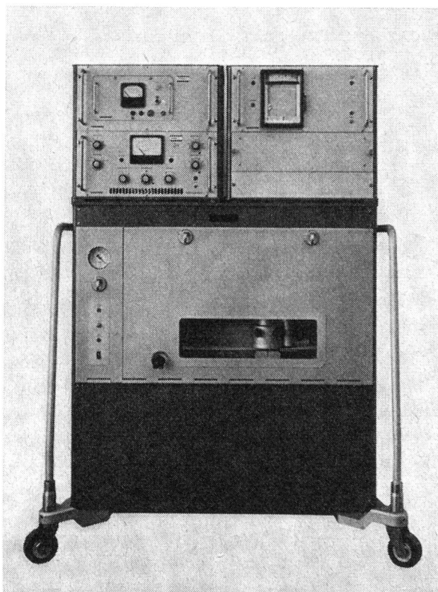
Abb. 2. Luftüberwachungsanlage (Detektor und Messeinheit)
