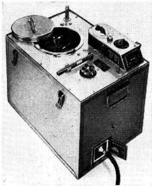
Der Densomat, das automatische Film- entwicklungsgerät.
