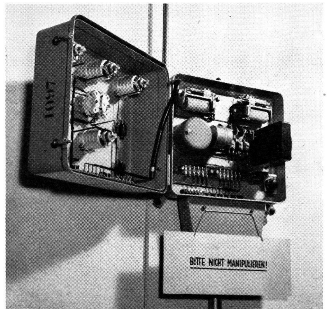
Hier die Innenansicht des Zusatzgerätes EXB 2, wie es, verbunden mit dem Ueberwachungsgerät, in einem Büro- oder Schutzraum montiert werden kann. Rechts aussen ist das Kontaktwerk sichtbar, das den Alarm erst nach drei in ununterbrochener Reihenfolge eingetroffenen Impulsen auslöst und damit jeden falschen Alarm ausschliesst.
