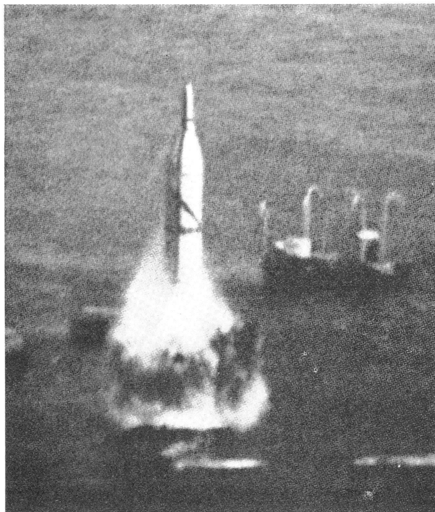
Polaris-Unterwasser-Abschussversuche in San Clemente, Californien
