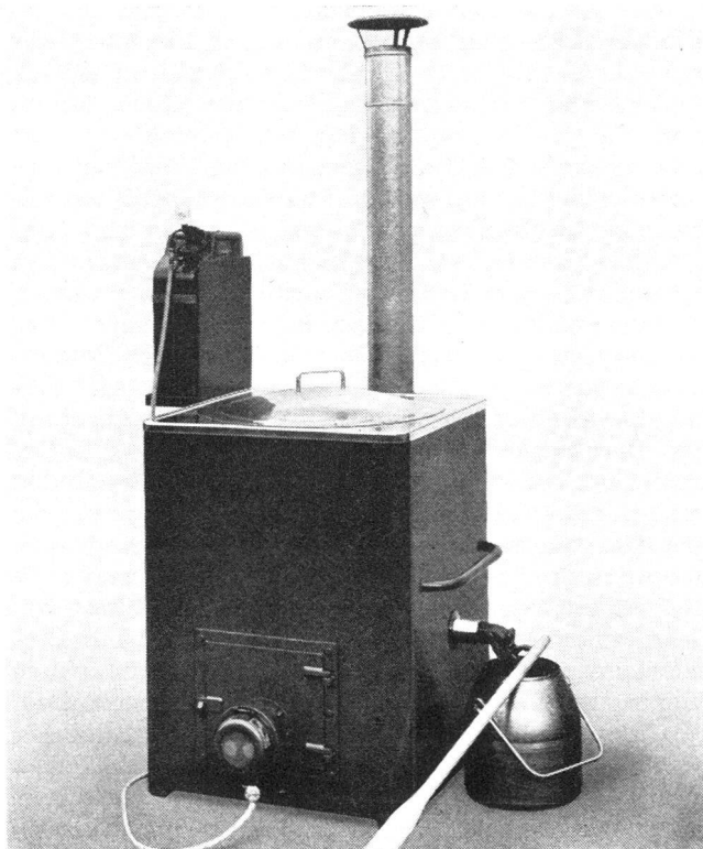
Kochkessel 150 Liter mit lose Deckel. Feuerung mit flüssigen oder festen Brennstoffen.
