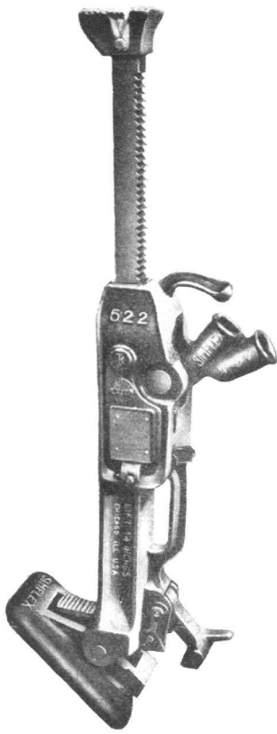
Universalwinde 5-20 t
