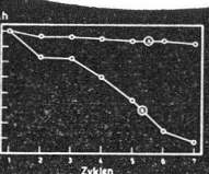
Fig. 10. Zyklusversuch mit Antimonhaltigem (A) und Antimonfreiem (B) Blei...
