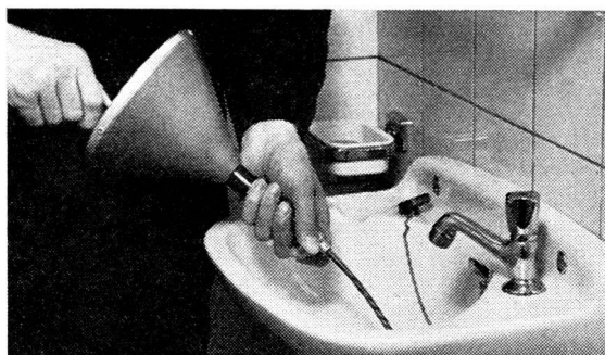
Entstopfer Typ D für Rohre von 15–50 mm \varnothing und bis zu 5 m Länge mit rostfreier Welle.
