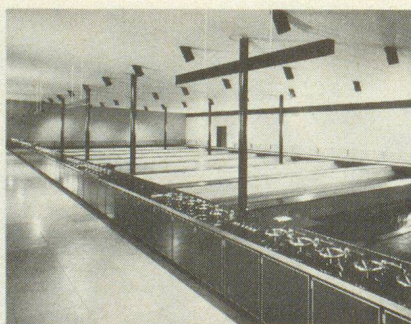
In Muttensz filtrieren Häny-Quarzsandfilter täglich rund 200 000 m 3 Wasser (Versorgungsgrundlage der Region Basel). Das Rohwasser wird dem Rhein entnommen, über offene Filter geleitet und zur Anreicherung des Grundwasserstromes im Hardwald zur Versickerung gebracht.
