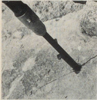
Fig. 25. Coin de clivage avec marteau de démolition A 7 dans la forure
