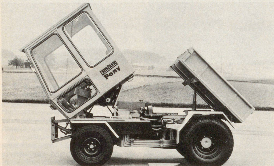
«Boschung-Pony» mit Rundblick-Sicherheitskabine nach vorne gekippt, ermöglicht unbehinderte Zugänglichkeit zu Motor, Getriebe und Aggregaten
