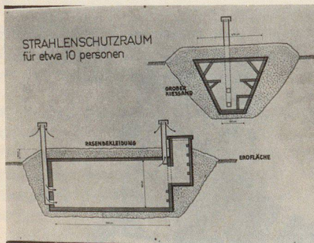
Planskizze eines Strahlenschutzraums auf dem Lande
