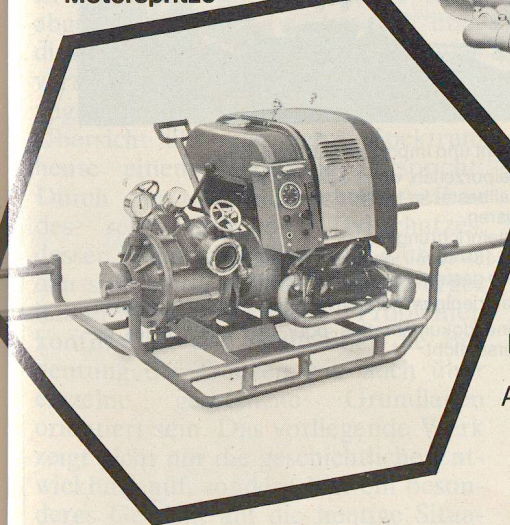
Motorspritze
