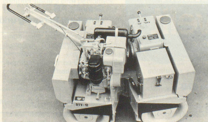
Knickgelenkte Tandem-Doppel- Vibrationswalze Ammann DTV-12 für universellen Einsatz von Schüttung bis Feinbelag. Gewicht: 900 kg.
