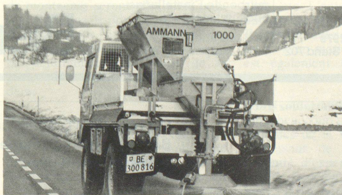
Aufsetzstreuer Ammann 1000 für Kommunalfahrzeuge Behälterinhalt 1 m 3 .
