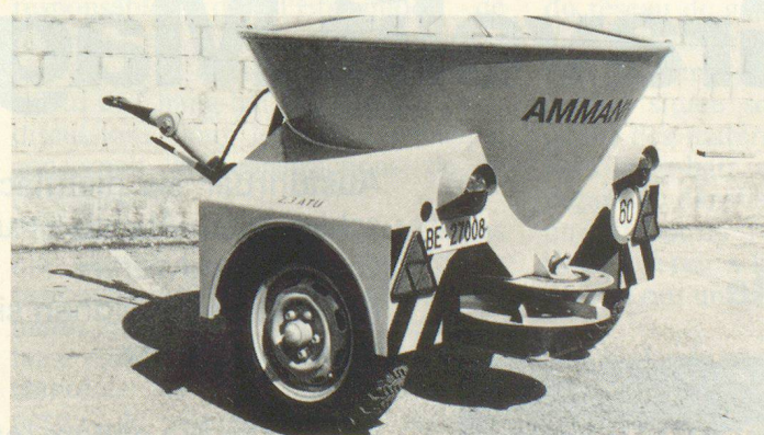
Anhängestreuer AMA 5F/FL Behälterinhalt 0,5 m 3 .
