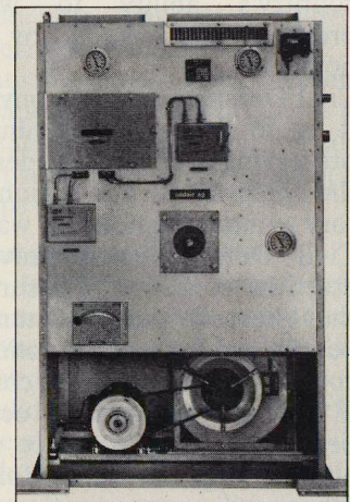
Belüftungsgeräte für Kommandoposten, Sanitätshilfsstellen, etc. Grössen VA 1200, 1800, 2400 und 4800. Diverse Spezialgeräte.
