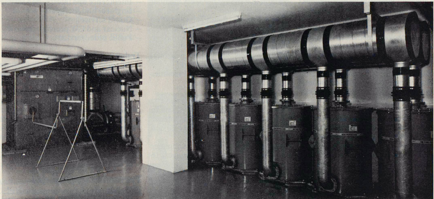
Ventilationsraum einer geschützten Operationsstelle. Filterluftmenge 4800 m 3 /h – Frischluftmenge 9600 m 3 /h.
