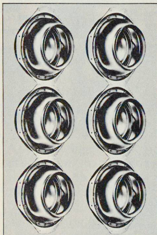
Explosions-Schutzventile für den druckfesten Abschluss von Zu- und Abluftöffnungen, 1 und 3 bar
