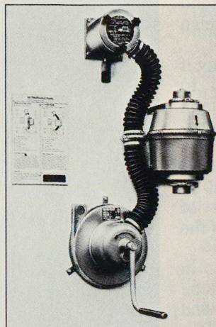
Belüftungsgeräte für den privaten Schutzraumbau Grössen VA 20, 40, 75 und 150
