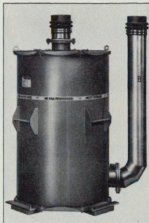
Gasfilter zum Schutz gegen chemische- und atomare Waffeneinwirkungen, Grössen GF 20, 40, 75, 150 und 600
