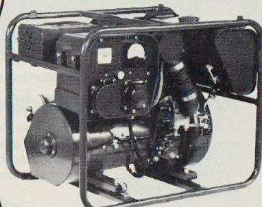
1200 W - 230 V
