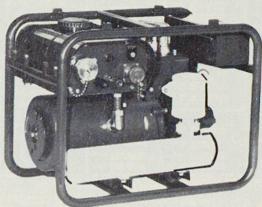
200 W - 12 V
