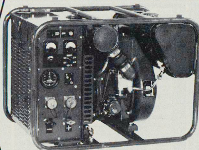
1200 W - 12/24 V
