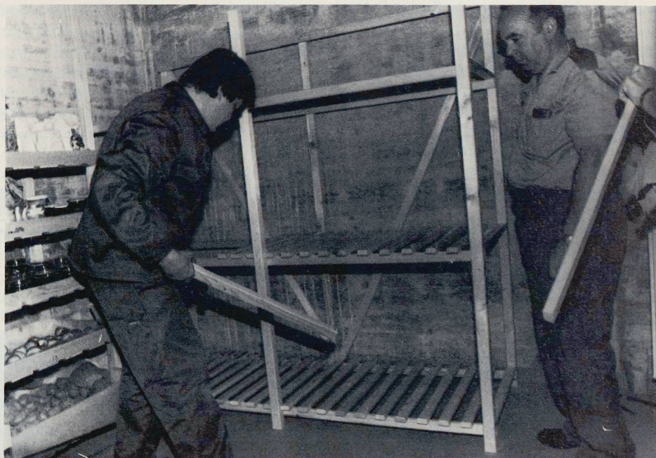
Beispiel der Liegestellen, wie sie in Steffisburg eingebaut werden. Die Dachlatten und Vierkanteleisten sind sauber glattgehobelt.
