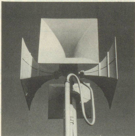
Schallstrahler einer Hochleistungssirene
