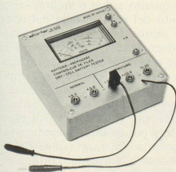
Batterie- prüfgerät BT 50410
