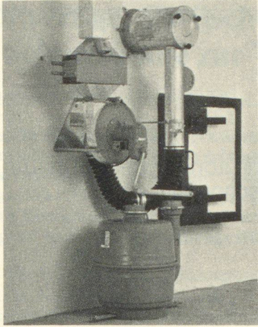
Schutzraumbelüftungsanlage mit Warmwasserlüfterhitzer.
