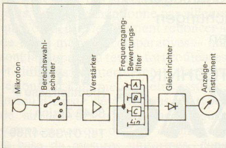
Abb. 1. Schallpegelmessgerät.
