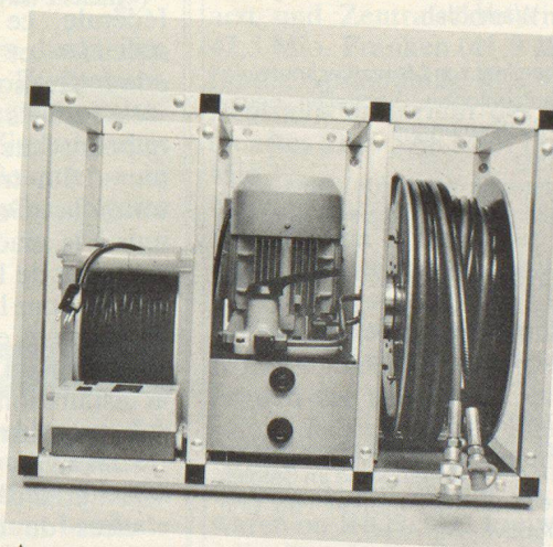
Antriebs einheiten
