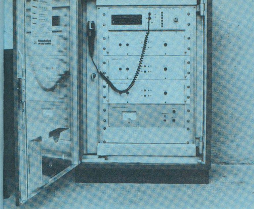
Elektronische Sirenanlage SES 130, 1500 W. Vollelektronisch, keine beweglichen Teile, dadurch wartungsfrei.
