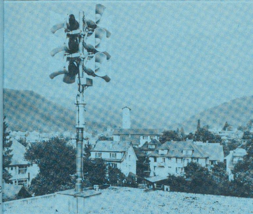
Sirenenmast mit 3 Lautsprecherebenen à 5 Lautsprecher, optmale, sektorielle Abstrahlung, witterungsbeständig und rostfrei.
