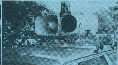
Mobile Sirenanlage für den schnellen, mobilen Einsatz. Vollelektronisch und mit Sprachdurchsage. Das Steuergerät hat im Handschuhfach platz, der Dachständer mit Lautsprecher und Drehleuchte ist blitzschnell montiert.
