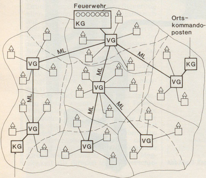
Abb./Fig.7 Autonome Anlage – Installation autonome Feuerwehr – Service du feu Ortskommandoposten – Poste de commandement local KG Kommandogerät – Appareil de commande VG Verteilgerät – Appareil de distribution Fernsteuergerät und Sirene – Appareil de télécommande et sirène ML Mietleitung – Ligne louée - Grenzen der technischen Alarmierungsbereiche – Limites des domaines d'alarme techniques --- Grenzen der Wirkungsbereiche – Limites des zones d'action
