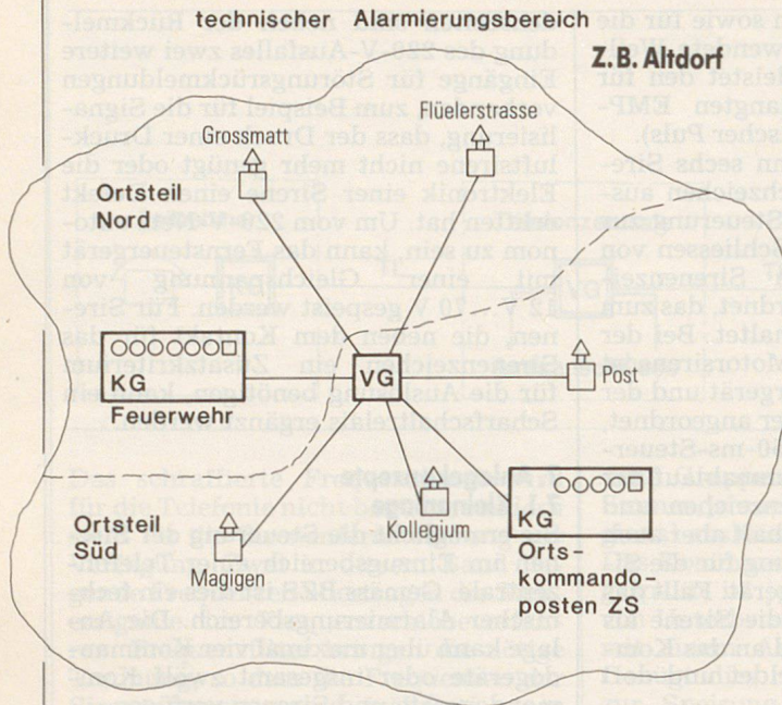
Abb./Fig.6 Kleinanlage – Petite installation Technischer Alarmierungsbereich – Domaine d'alarme technique Ortsteil Nord – Quartiers nord Feuerwehr – Service du feu Ortsteil Süd – Quartiers sud Ortskommandoposten ZS – Poste de commandement local PC KG Kommandogerät – Appareil de commande VG Verteilgerät – Appareil de distribution Fernsteuergerät und Sirene – Appareil de télécommande et sirène
