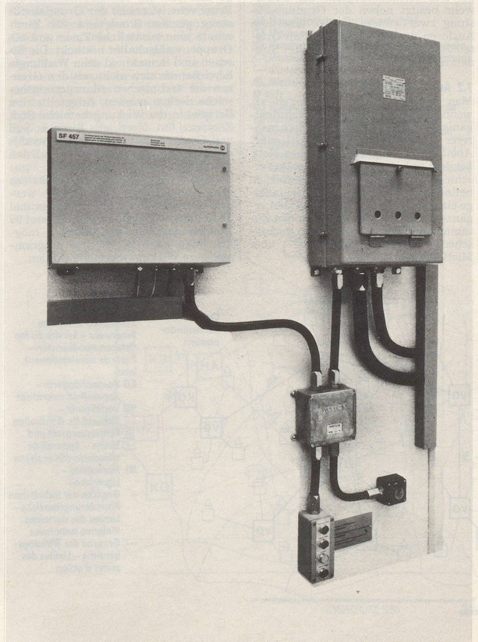
Abb./Fig. 4 Verteilgerät – Appareil de distribution Von übergeordnetem VG – D'un appareil de distribution hiérarchiquement supérieur Zu SMT 75 – Vers l'installation SMT 75 Zu untergeordnetem VG – Vers un appareil de distribution hiérarchiquement subordonné KG Kommandogerät – Appareil de commande FG Fernsteuergerät – Appareil de télécommande VG Verteilgerät – Appareil de distribution
