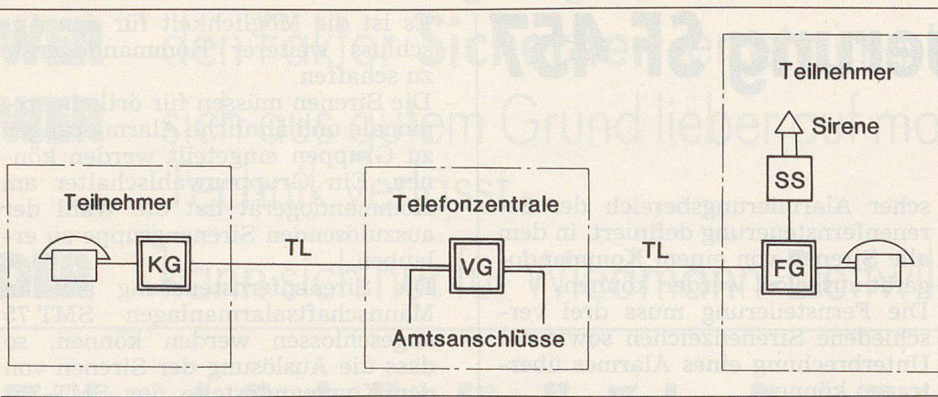
Abb./Fig. 1 Funktionsprinzip der Sirenenfernsteuerung – Principe de fonctionnement de la télécommande de sirènes Teilnehmer – Abonné Telefonzentrale – Centrale téléphonique Amtsanschlüsse – Raccordements réseau Sirene – Sirène KG Kommandogerät – Appareil de commande VG Verteilgerät – Appareil de distribution FG Fernsteuergerät – Appareil de télécommande SS Sirenschalter – Commutateur de sirène TL Teilnehmerleitung – Ligne d’abonné □ Anlagenteile der Sirenenfernsteuerung – Parties d’installation de la télécommande des sirènes
