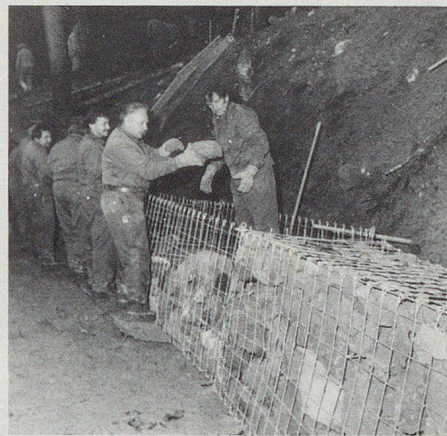
Drahtschotterkörbe werden gefüllt, um eine Böschung rutschsicher zu gestalten.
