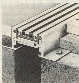
DEFLEX-Dehnfugenelement – mit diesen Dilatationsfugensystemen werden die äusserst schädlichen Schwundrisse bei befestigten Bauten und Anlagen vermieden.
